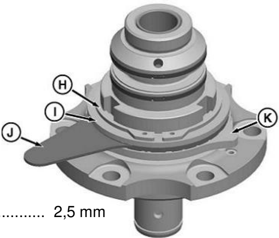
H—Circlip I—Plateau de pression extérieur J—Disque de friction K—Plaque intérieure d'actionnement de frein de prise de force
