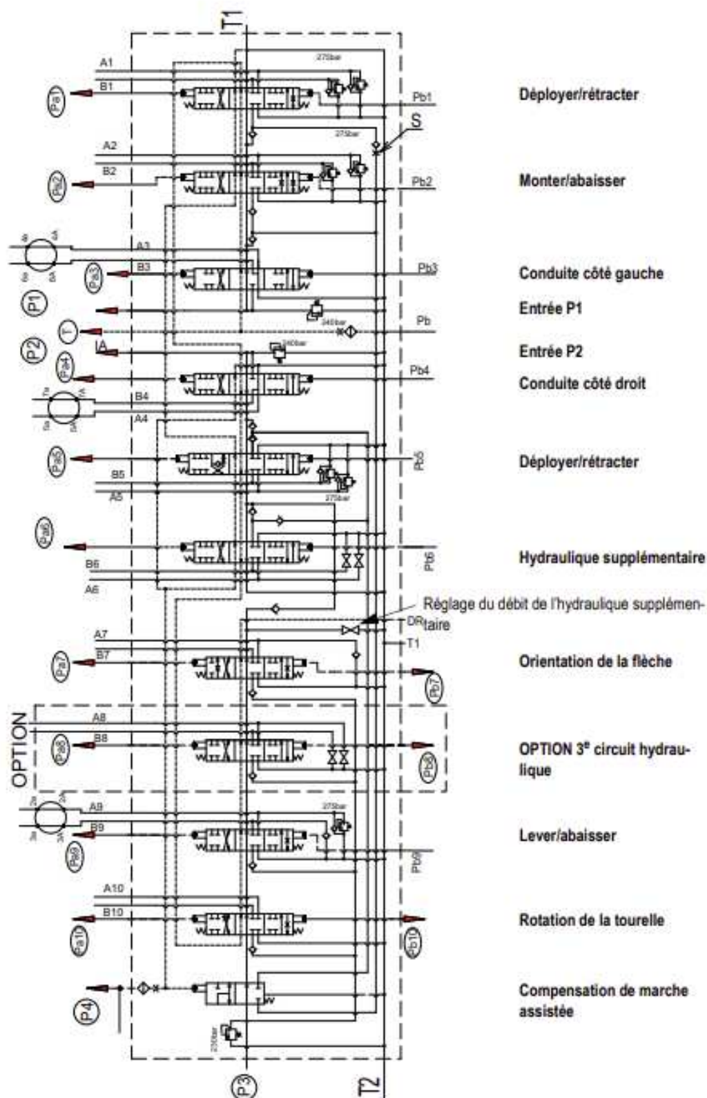
Schéma du bloc de commande mobile
