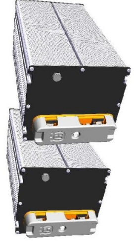
MODULE DE BATTERIES | 4 kWh (2x2 kWh) Batteries au lithium afin d'optimiser les performances et la durée de vie.
