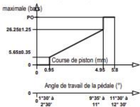
Courbe caractéristique du clapet de conduite
