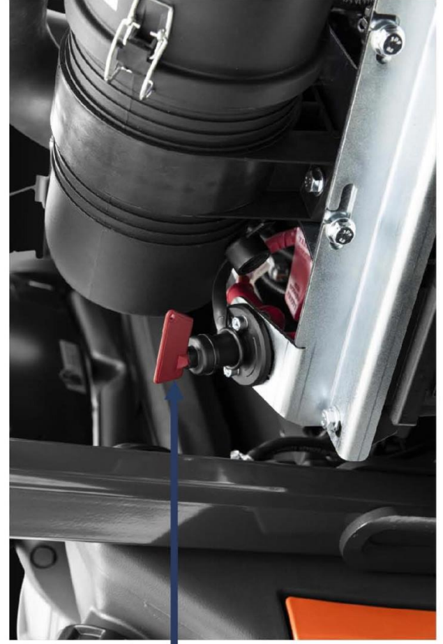
Coupe circuit, 12 V
