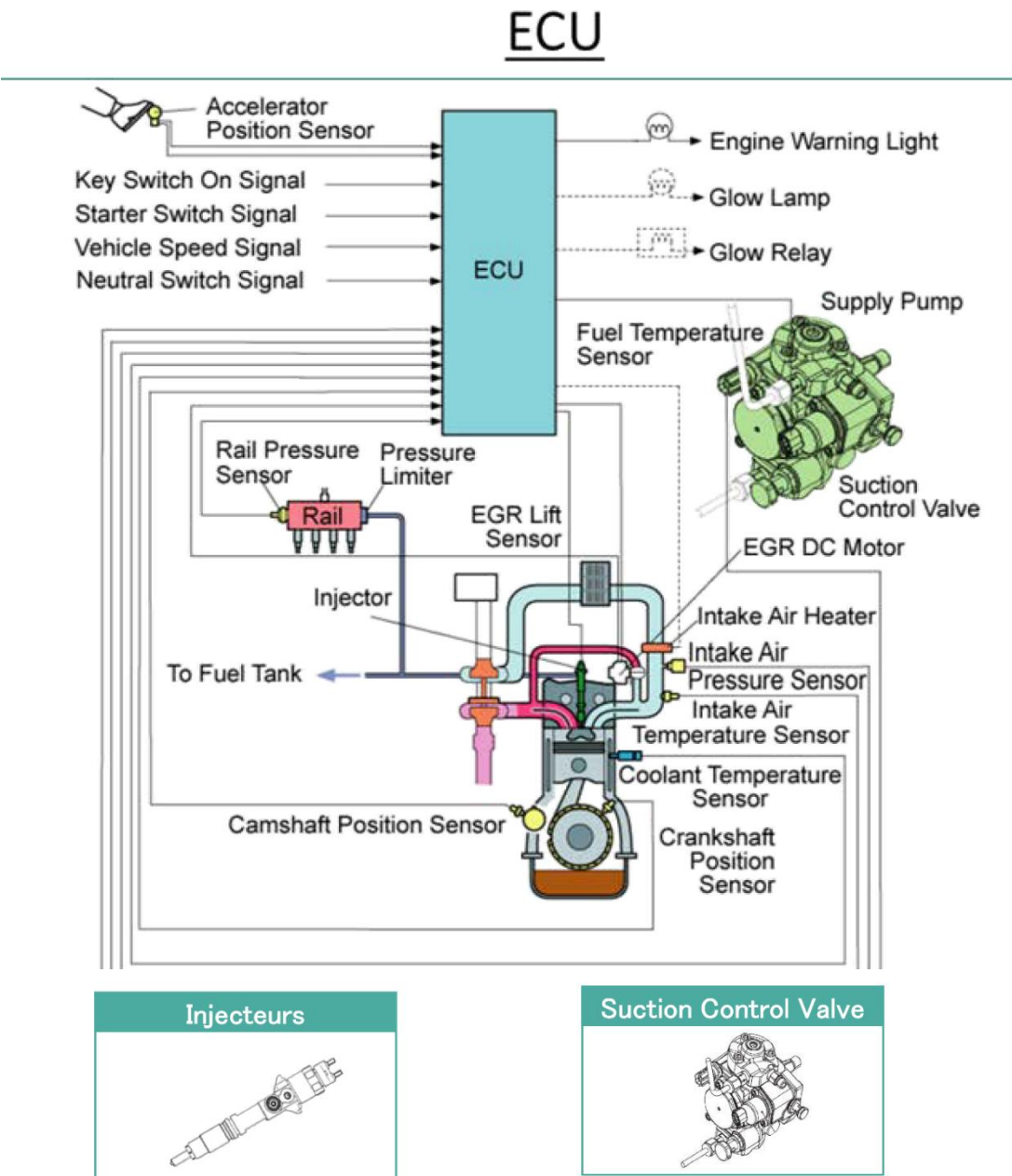
Exemple d'actionneurs
