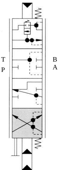
Fig.24 Tiroir de basculement en position d'abaissement
