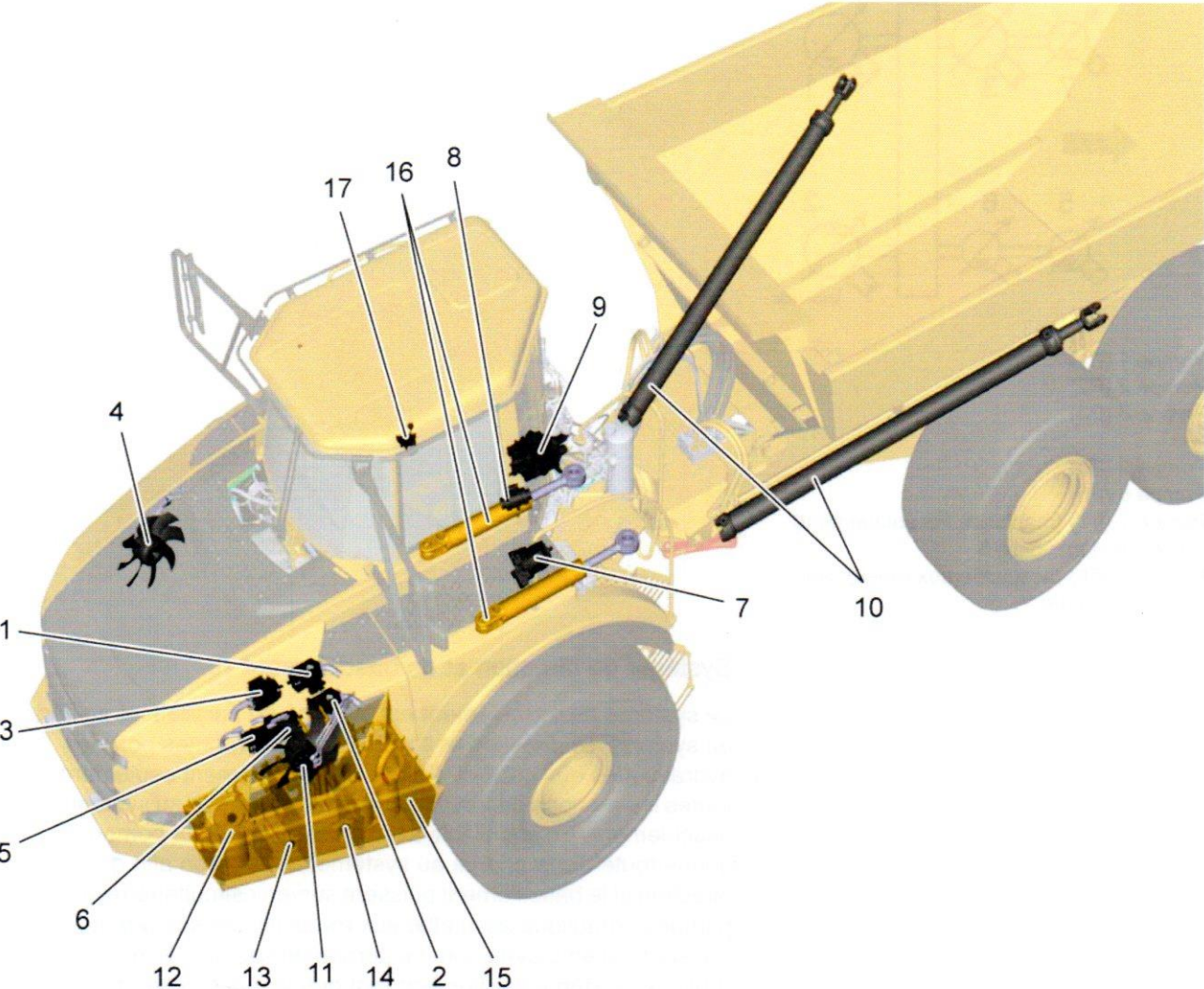
Fig.2 1 Pompe 1 (P1) 2 Pompe 2 (P2) 3 Pompe 3 (P3) 4 Moteur de ventilateur, radiateur d'eau 5 Pompe 5 (P5) 6 Pompe 6 (P6) 7 Pompe 8 (P8) 8 Vérin amortisseur 9 Distributeur de direction et de basculement 10 Vérin de basculement 11 Moteur de ventilateur du refroidisseur d'air de suralimentation 12 Réservoir, huile de refroidissement des freins 13 Voyant de contrôle de niveau de liquide de frein 14 Regard vitré, huile hydraulique 15 Réservoir, huile hydraulique 16 Vérin de direction 17 Vanne PWM (vanne de pression d'assistance) de basculement
