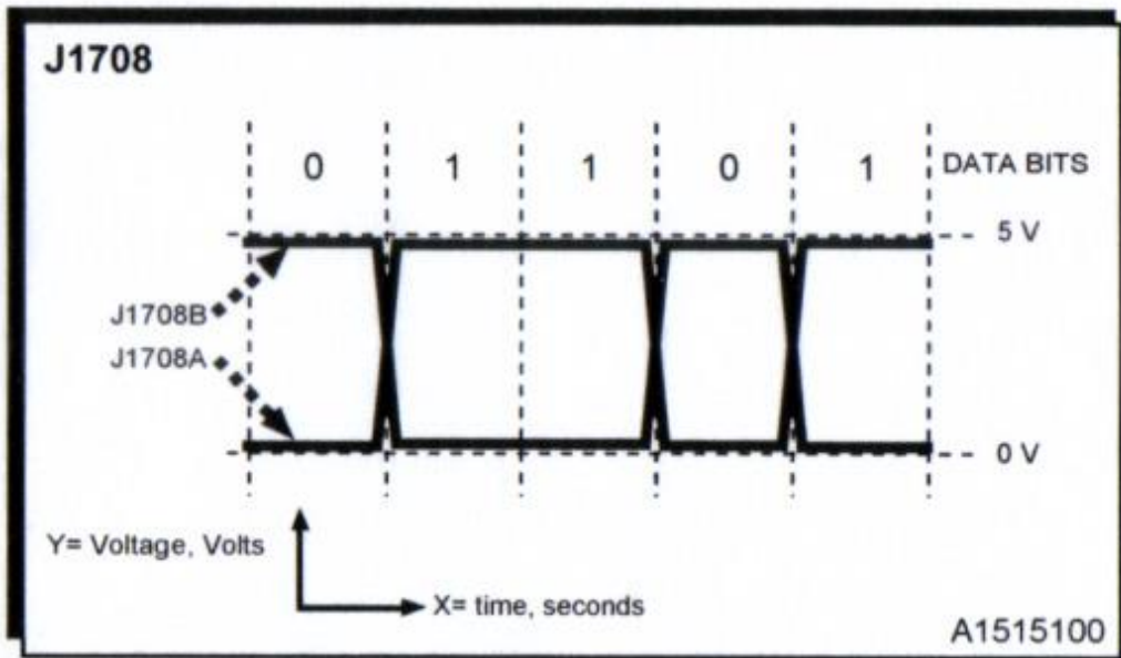
Niveaux de tension bus J1708
