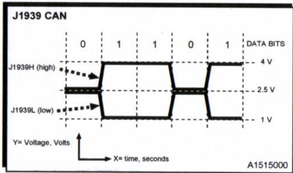
Niveaux de tension bus CAN J1939
