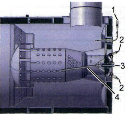
Vue détaillée du brûleur
